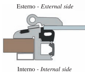
Profilo apribile solo vetro - Openable profile - glass only
