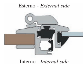
Profilo apribile con telaio - Openable profile with frame
