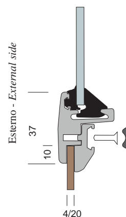
Profilo fisso Fixed profile
